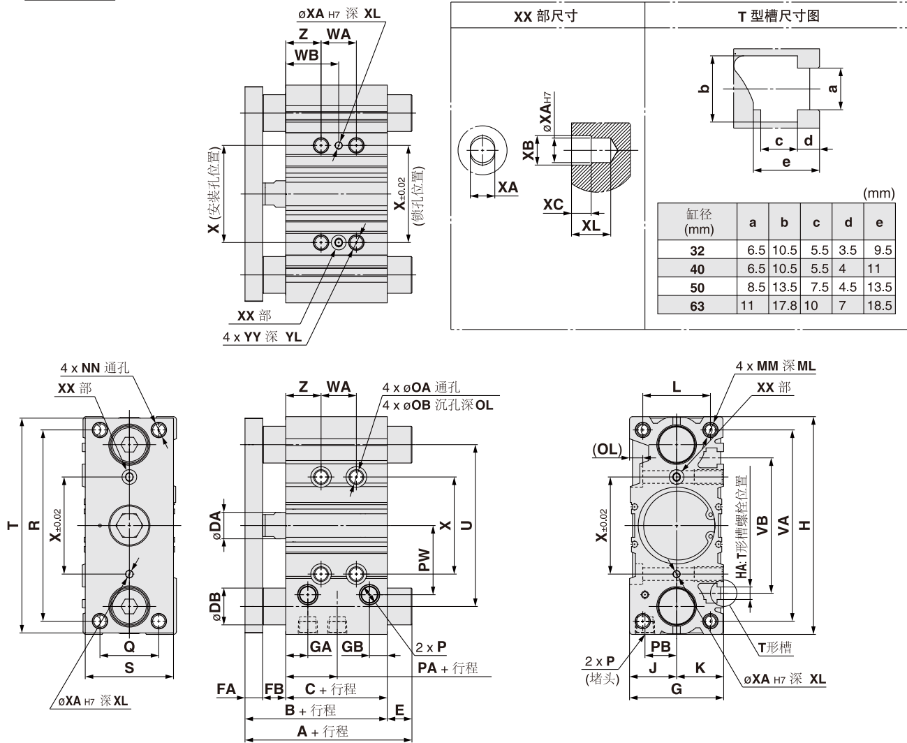
外形尺寸图（毫米）
